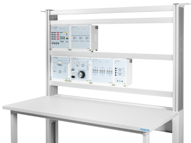
Conjunto de equipos TP 8015-2
