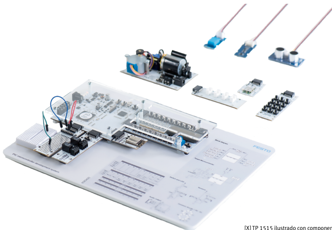
[X] TP 1515 ilustrado con componentes opcionales
