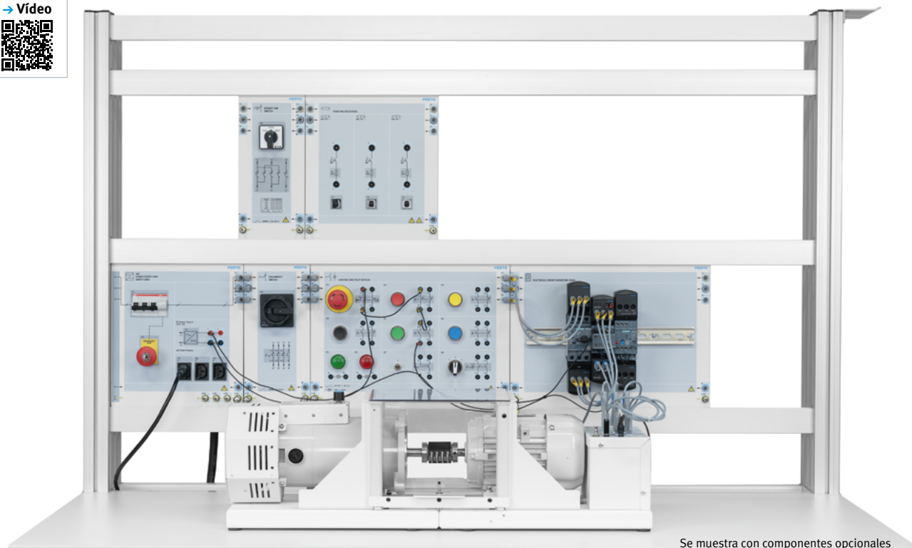
Se muestra con componentes opcionales
