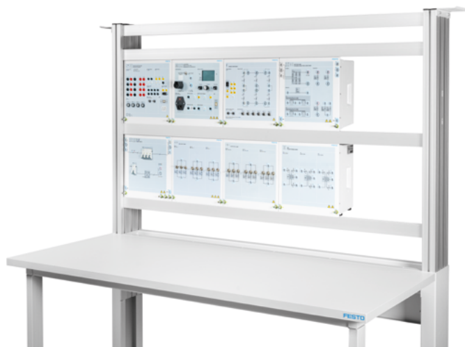
Conjunto de equipos TP 8015-5
