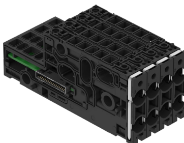
Gruppe von Einzelscheiben mit jeweils einteiliger Leiterplatte
