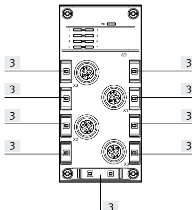
[3] Platz für Bezeichnungsschild
