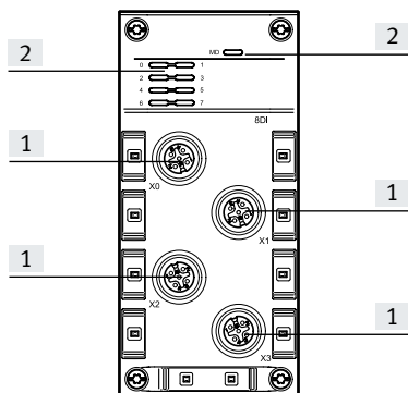
[1] Elektrischer Anschluss Eingänge [2] LED-Anzeigen
