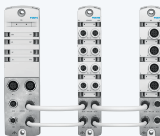
Decentralized remote I/O modules CPX-AP-I
