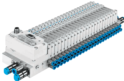
Unità di valvole VTUG plug-in
