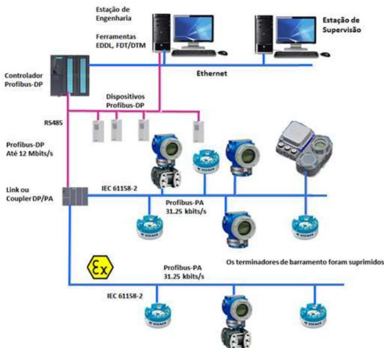
Figura 3.9-1- Ligação de um equipamento Profibus PA no barramento
