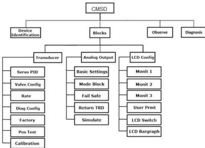
Figura 4.5-1 - Árvore de programação do CMSD PROFIBUS
