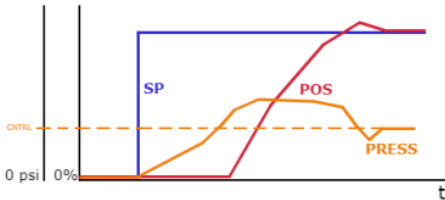
Figura 4.9-2 – Setpoint, Posição e Pressão
