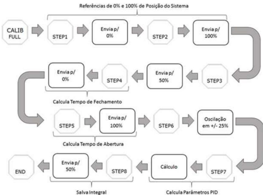
Figura 4.6-3 - Diagrama de passos da auto calibração completa.
