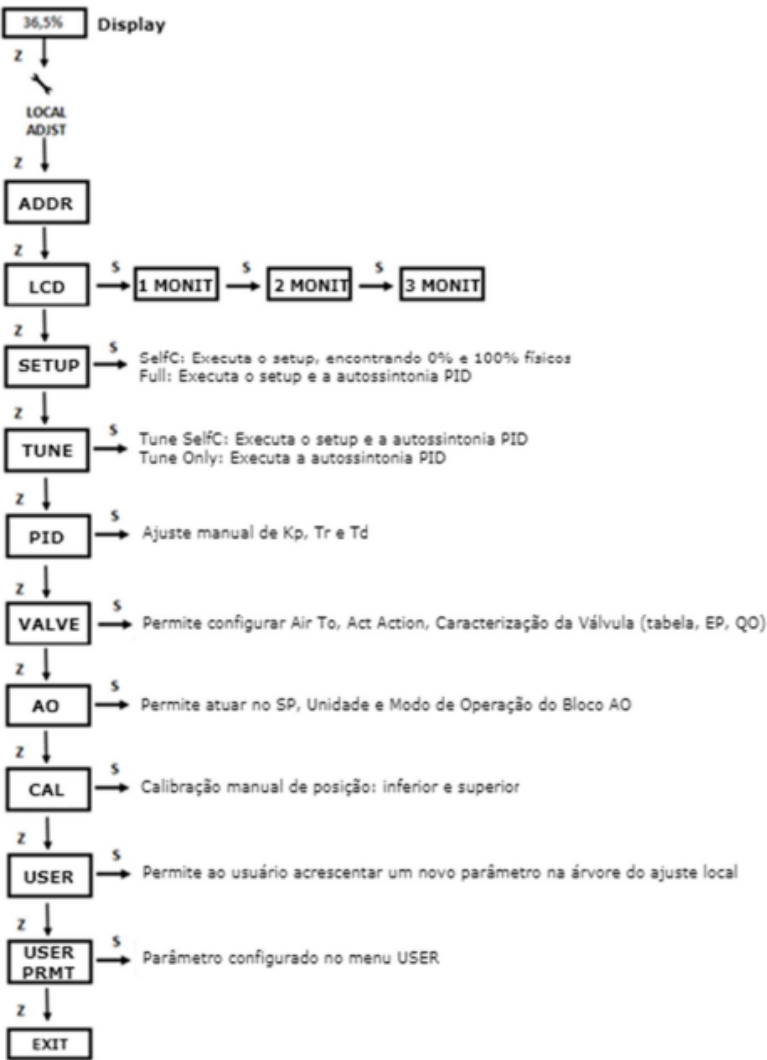
Figura 4.4-1 – Árvore de programação do ajuste local
