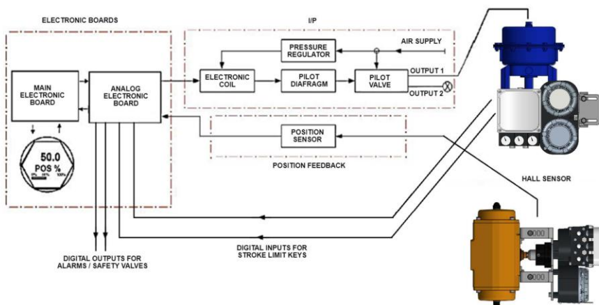
Figura 2.1-1 Diagrama de blocos do CMSD Profibus.
