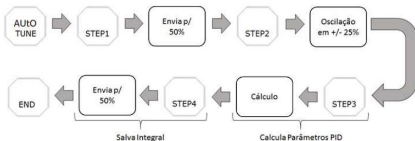
Figura 4.6-2 - Diagrama de passos da autossintonia do controle PID
