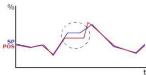
Figura 4.9-3 – Setpoint e posição emperramento intermediário.
