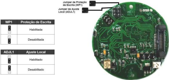
Figura 4.2-1 – Detalhe da placa principal com jumpers
