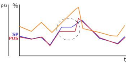
Figura 4.9-4 – Setpoint, posição e pressão emperramento intermediário.
