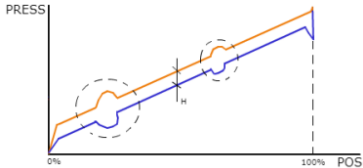
Figura 4.9-5 – Posição e pressão e emperramento.
