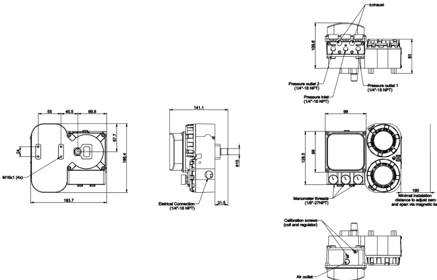
Figura 3.5-2- Dimensional Externo
