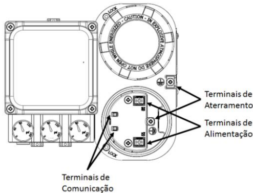
3.6-2 –Terminais elétricos de ligação e tabela para a versão de sensor magnético
