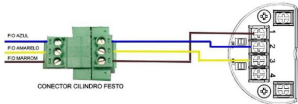
3.6-3 –Terminais elétricos de ligação régua potenciometrica
