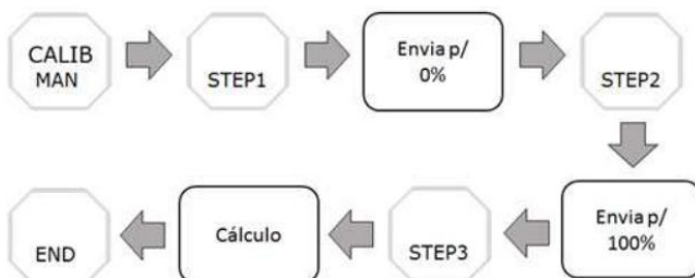
Figura 4.6-4 - Diagrama de passos da calibração manual de posição.
