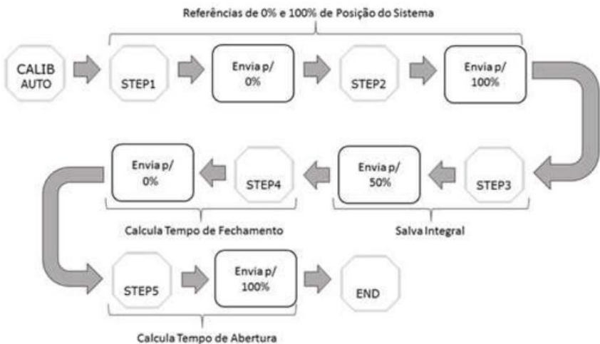
Figura 4.6-1 Diagrama de passos da calibração automática de posição.
