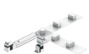
Transfer mit dem Elektrozylinder EPCS und Drehantrieb ERMS
